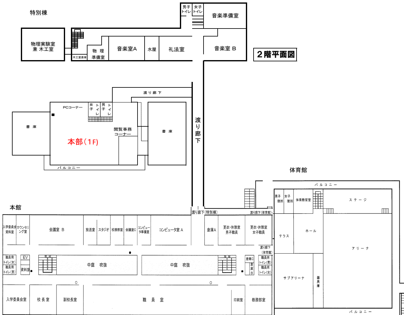
2階平面図
